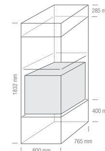
Dimensions extérieures
