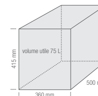
Dimensions intérieures
